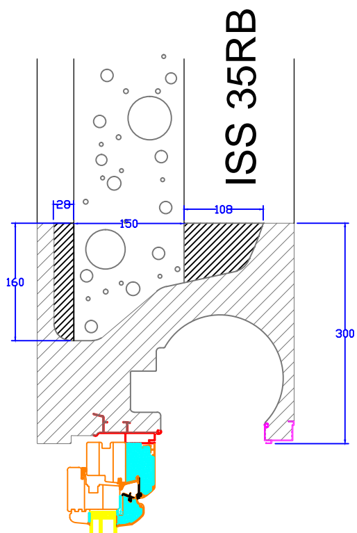
B-REKORD 35 ( 38-ból vágott) kitakart betoncsatornával
